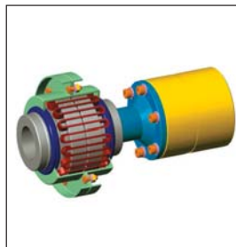
T.TL.NPE Spacer type
